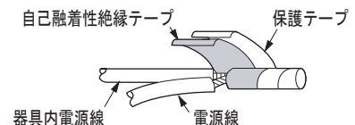
電源線接続のしかた(図4)
