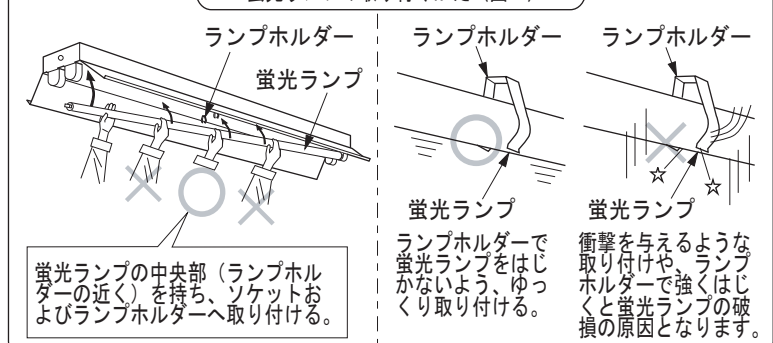
蛍光ランプの取り付けかた(図5)
