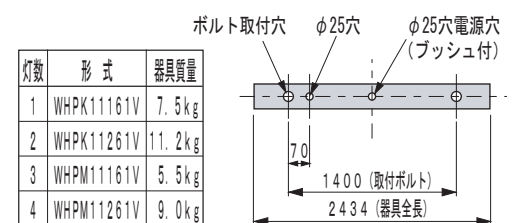
器具質量と背面取付穴(図2)
