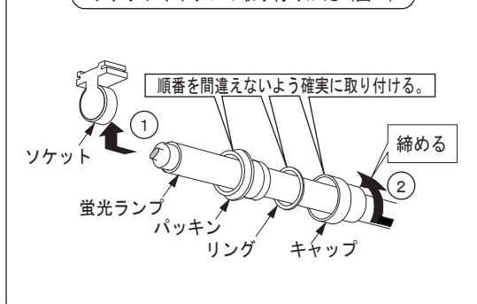
ソケットキャップの取り付けかた(図6)
